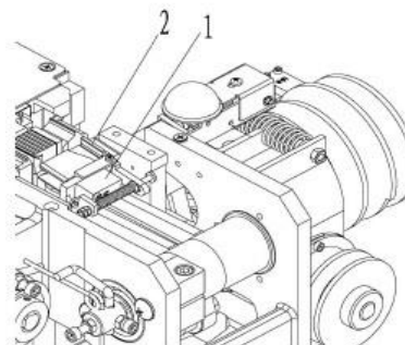
1. Выключатель LS5 2. Рычаг
