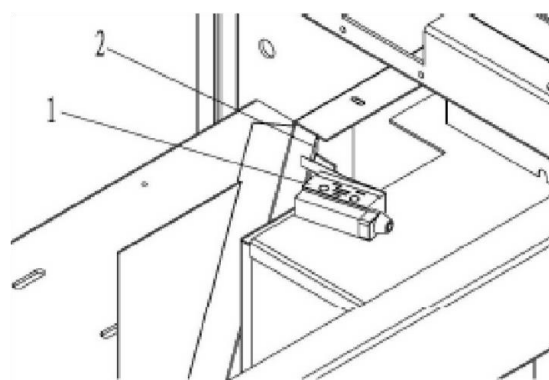
1. Выключатель LS7 2. Дверца
