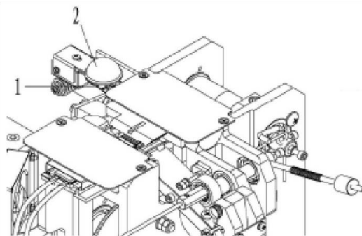
1. Выключатель LS6 2. Шаровой переключатель
